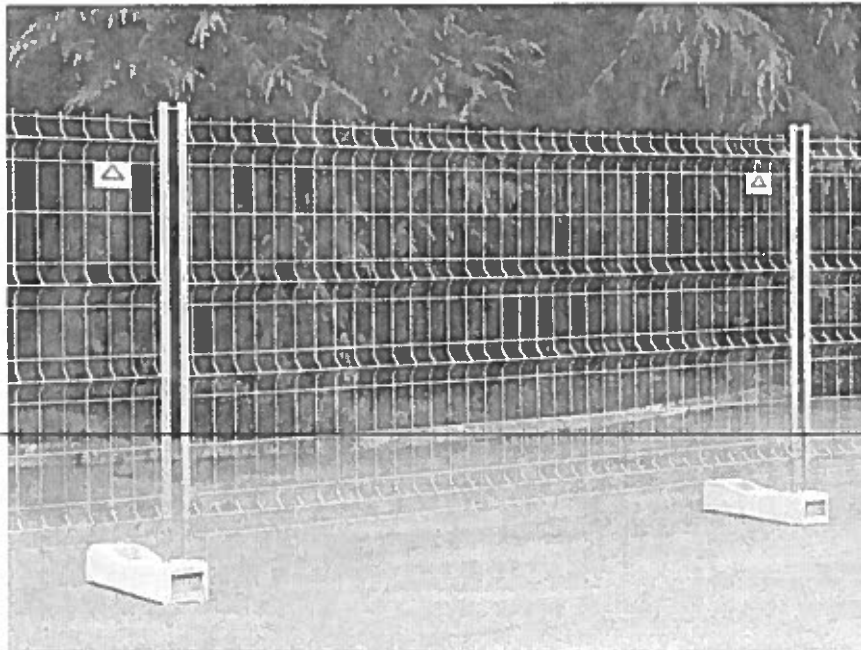
Figura 2: Modulo Recinzione Temporanea dotata di CERTIFICAZIONE STATICA (dim 3,00*2,00) - Fili orizzontali e verticali: 3,2mm - Maglia 100*300mm - Tubo orizzontale: diametro 30mm - Tubo verticale: diametro 40mm - completo di elementi di zavorra in cls - vibrato di adeguato peso.
