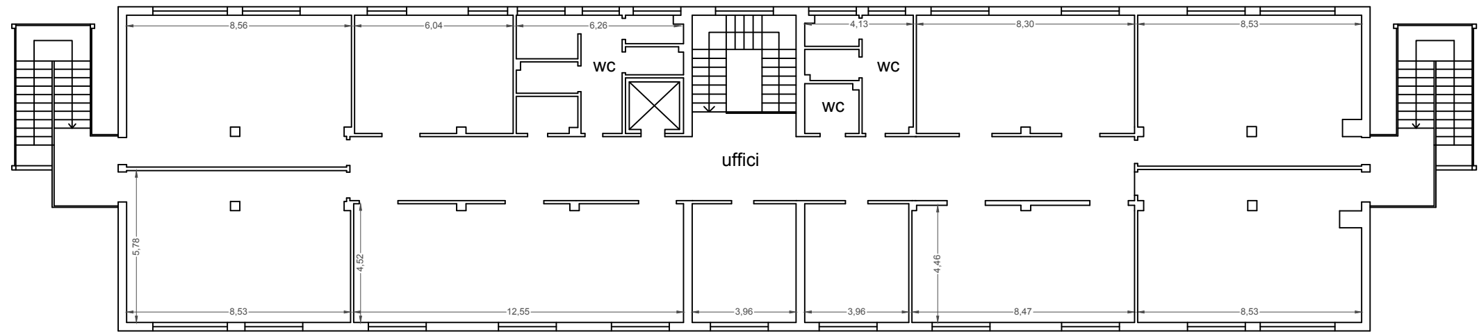
PIANO PRIMO
