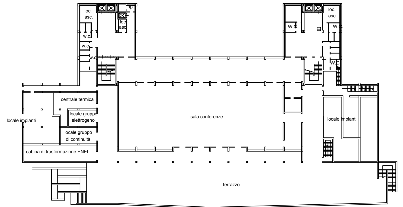
SOPPALCO SEMINTERRATO
