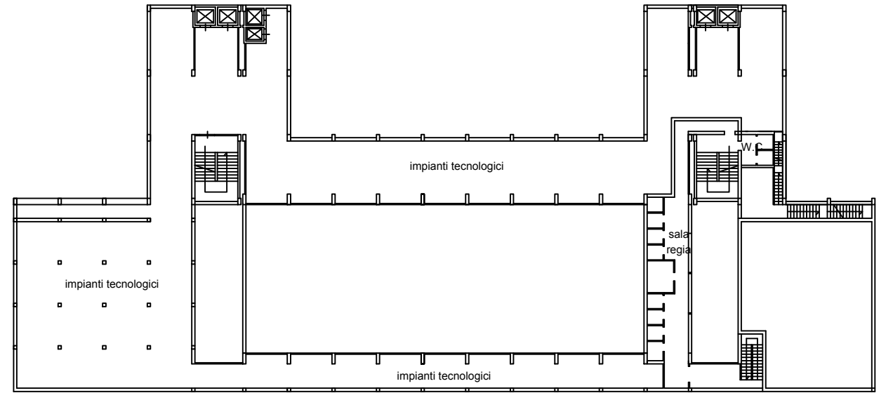
SOPPALCO SEMINTERRATO
