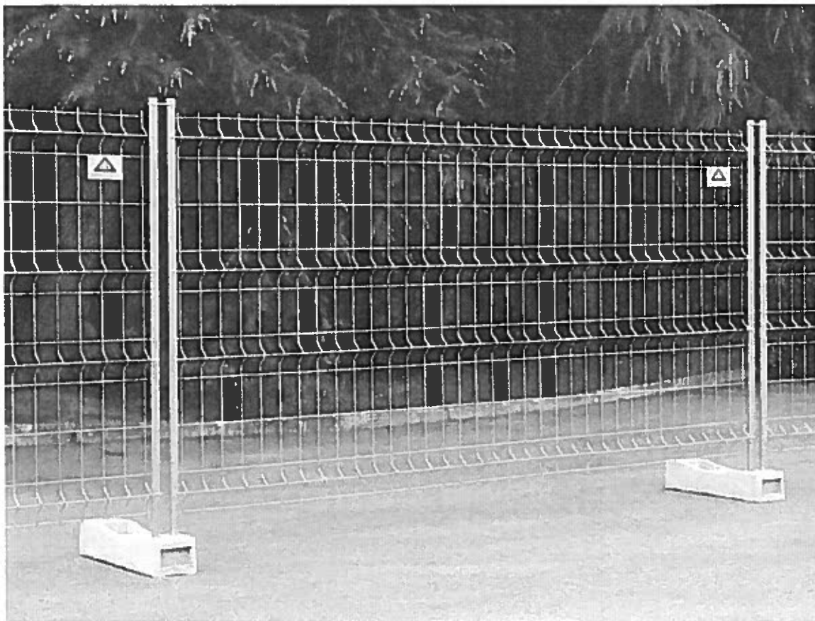
Figura 2: Modulo Recinzione Temporanea dotata di CERTIFICAZIONE STATICA (dim 3,00*2,00) - Fili orizzontali e verticali: 3,2mm - Maglia 100*300mm - Tubo orizzontale: diametro 30mm - Tubo verticale: diametro 40mm - completo di elementi di zavorra in cls - vibrato di adeguato peso.
